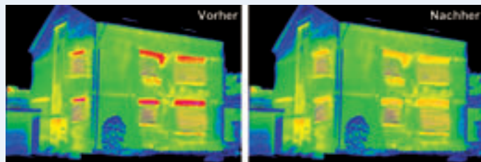
Auf den Wärmebildern ist erkennbar, dass über ungedämmte Rollladenkästen viel Energie verloren geht. Mit einer nachträglichen Dämmung lassen sich die Wärmeverluste um 60 Prozent reduzieren. Fotos: Selit/rbr
